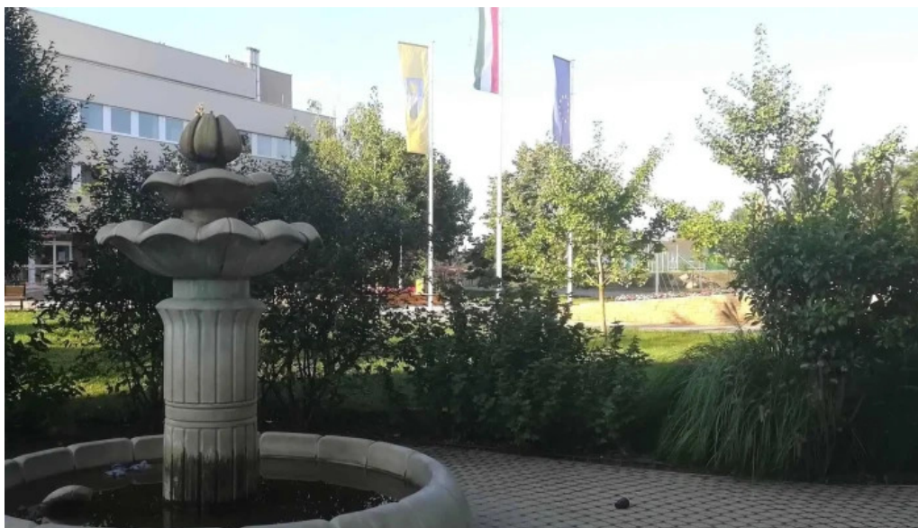
Kormanyablak weboldal
